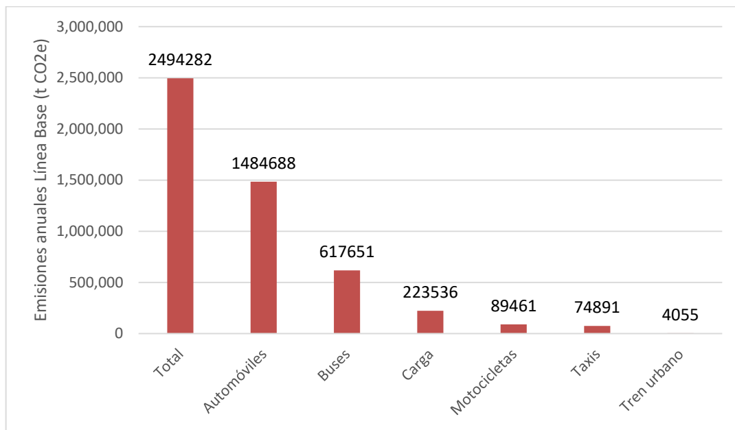
Figura 12. Emisiones anuales de Línea Base WTW del Sector Transporte de la GAM en t CO 2 e (incluyendo BC), emisiones absolutas totales y por modo de transporte (2014).
